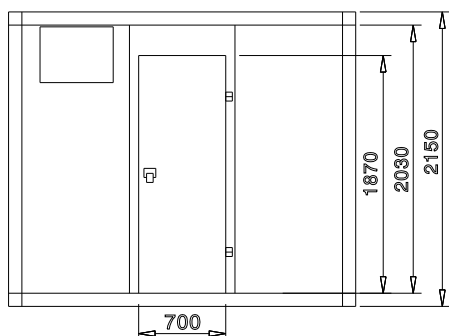
Fronte
